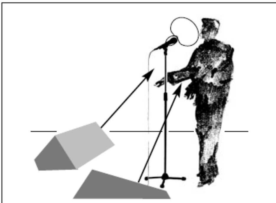
(A mikronos ideális elhelyezése, maximális gain-nél, még gerjedés nélkül.)
